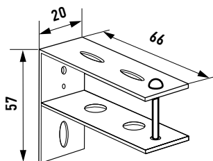
Установочный кронштейн 245780
