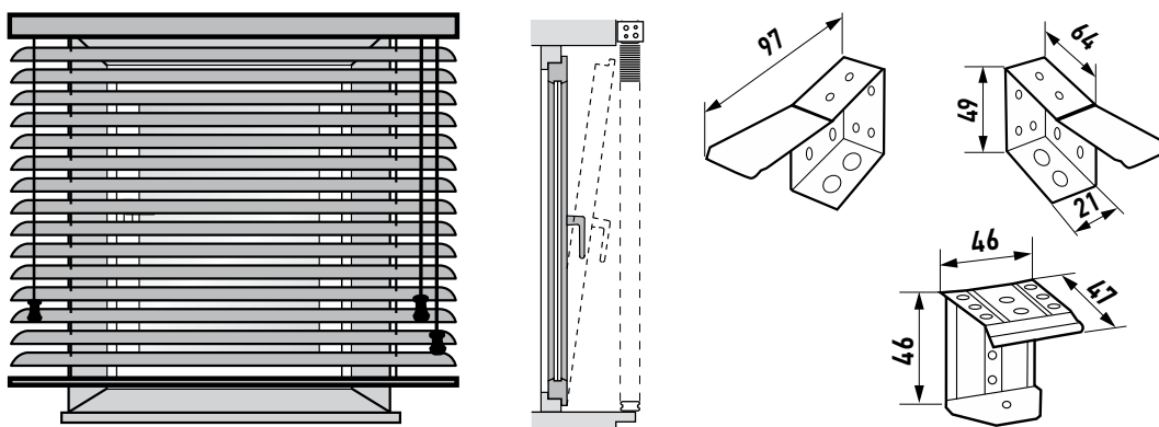
Комплект стандартных кронштейнов-пара боковых (245581)+центральный кронштейн (245580)
